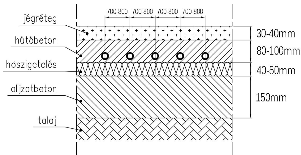
Normál pályatest rétegrendje
